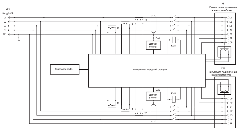
Рис.1. Структурная схема и схема подключения ЗС
