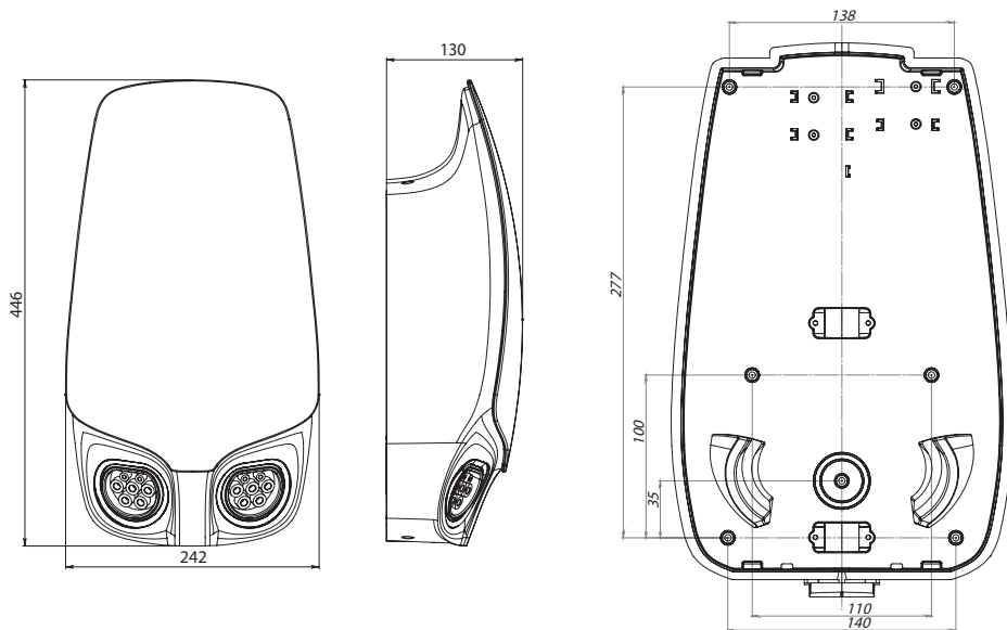
Рис.2. Габаритный чертеж
